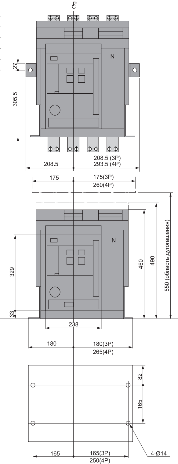
Монтажные отверстия
