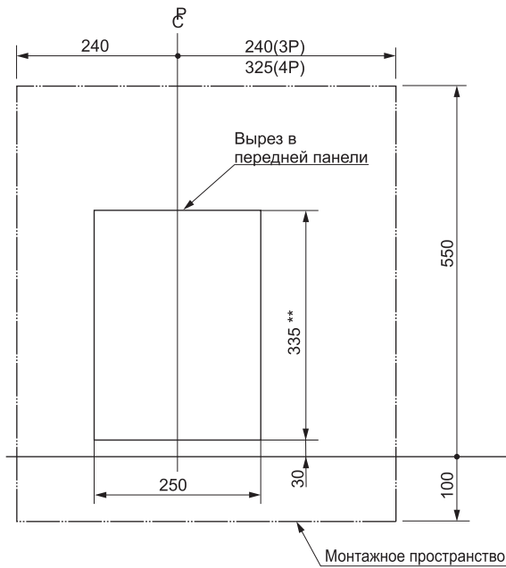
Вырез панели
