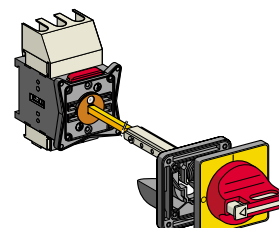
Монтаж на заднюю панель шкафа
