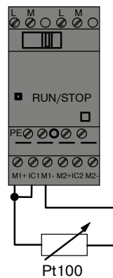
2-проводная схема
