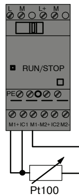
3-проводная схема
