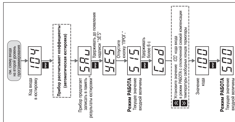
Схема П4.2. Последовательность действий при юстировке прибора с термопарой
